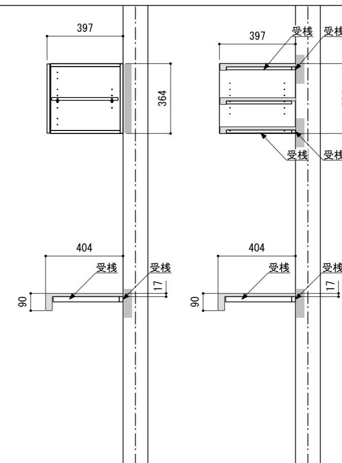
A-A' 断面
