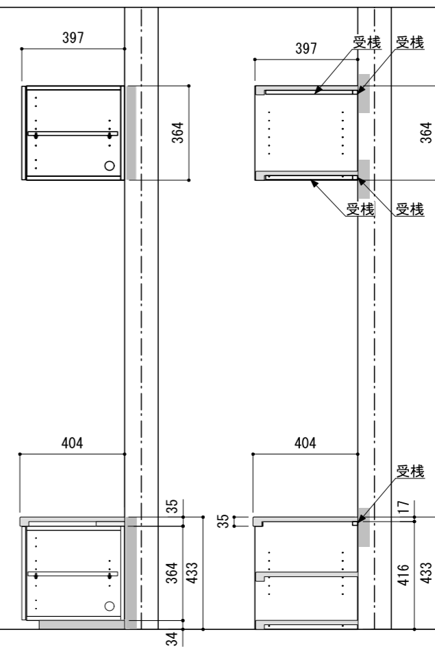
A-A' 断面
