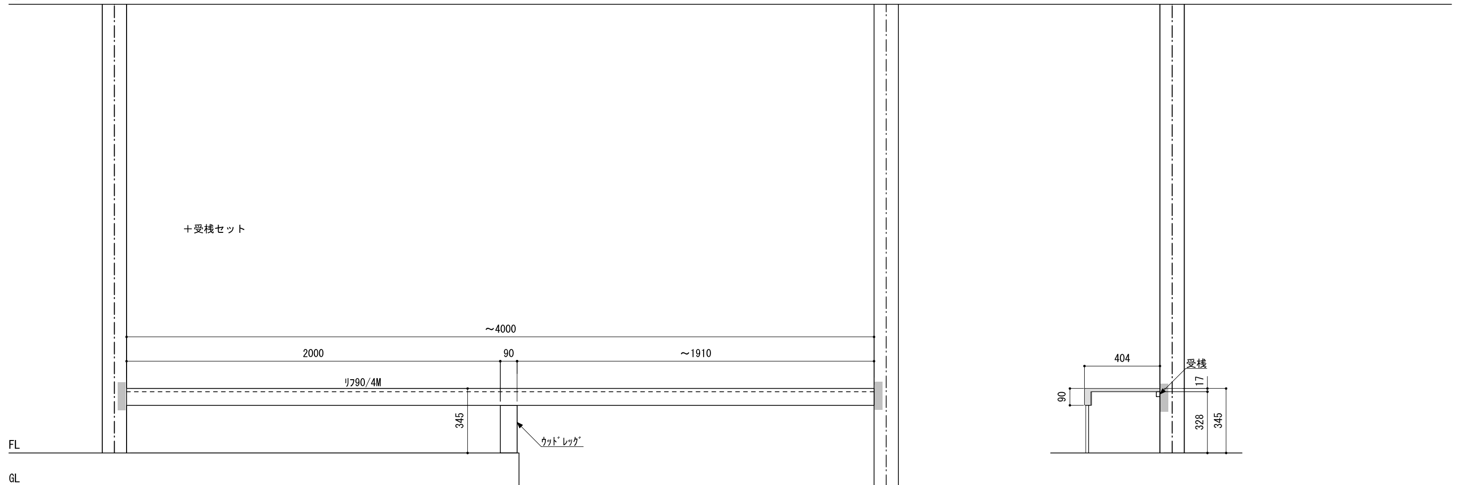
A-A' 断面
