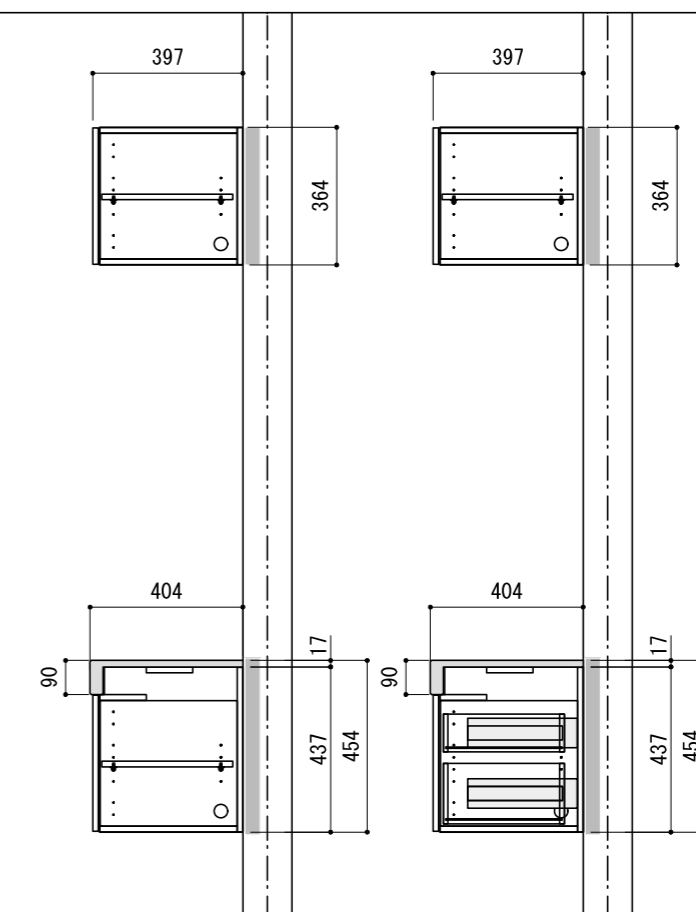
A-A' 断面
