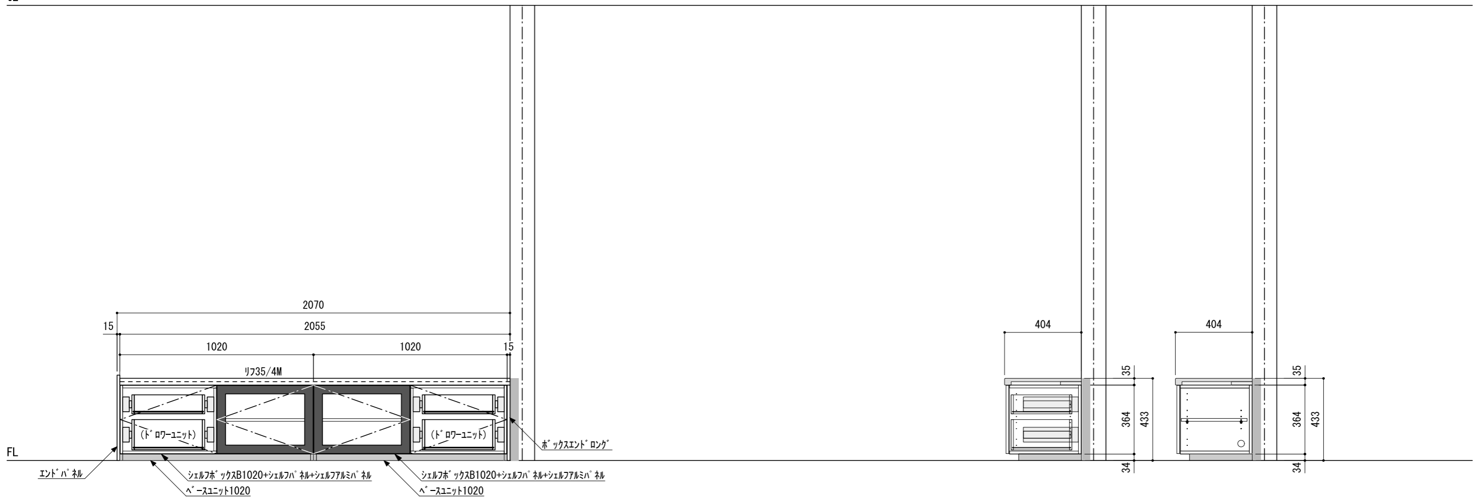
A-A' 断面
