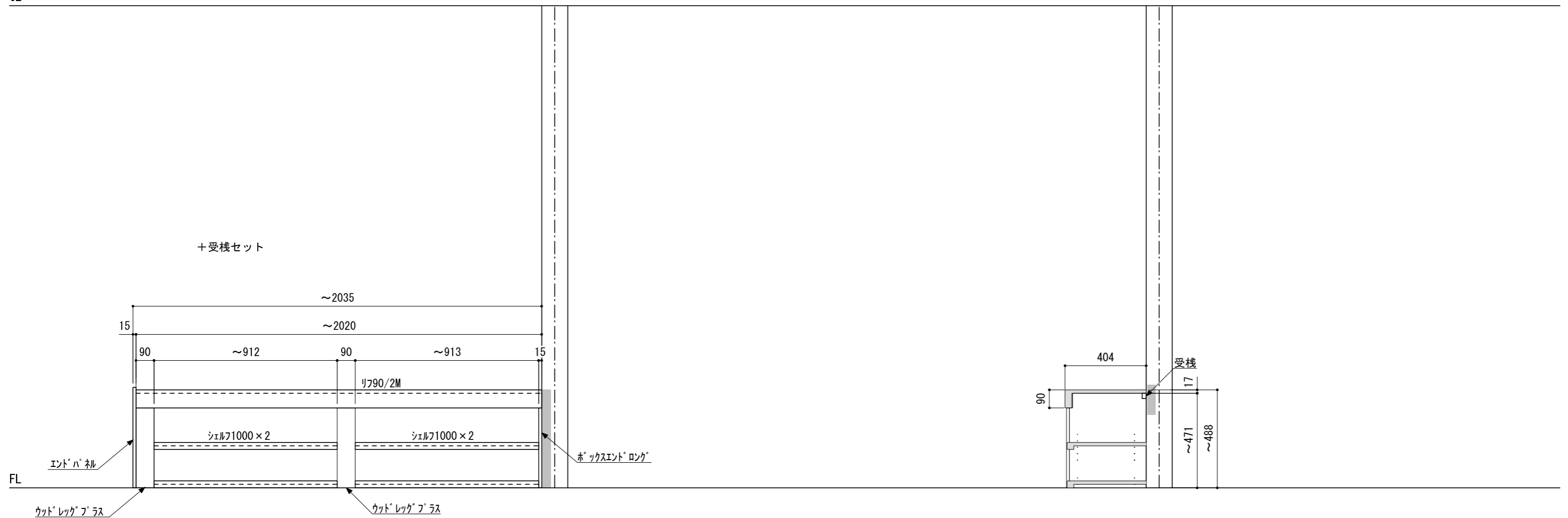
A-A' 断面
