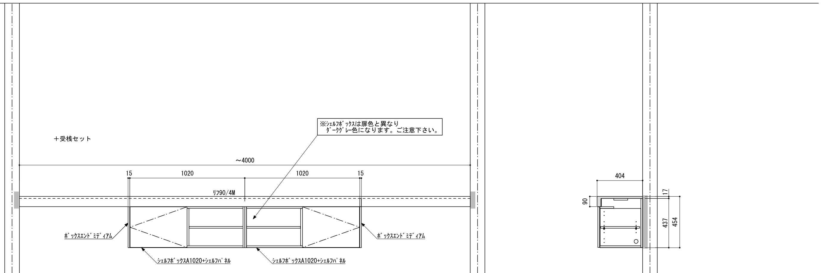
A-A' 断面
