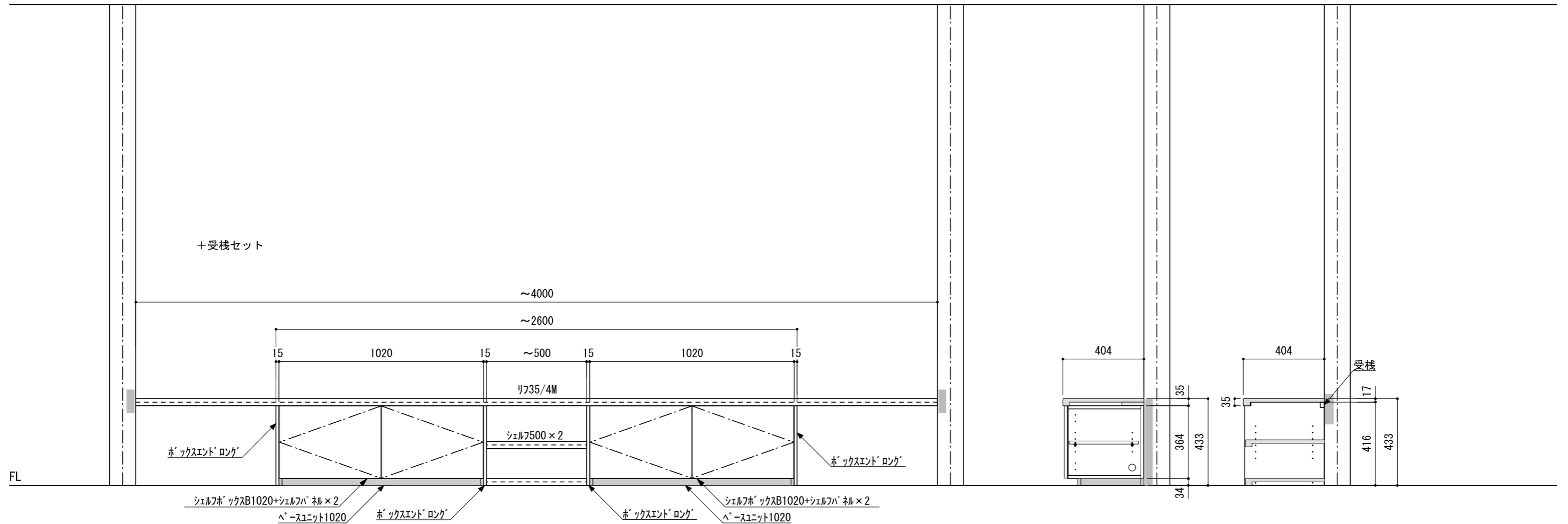
A-A' 断面
