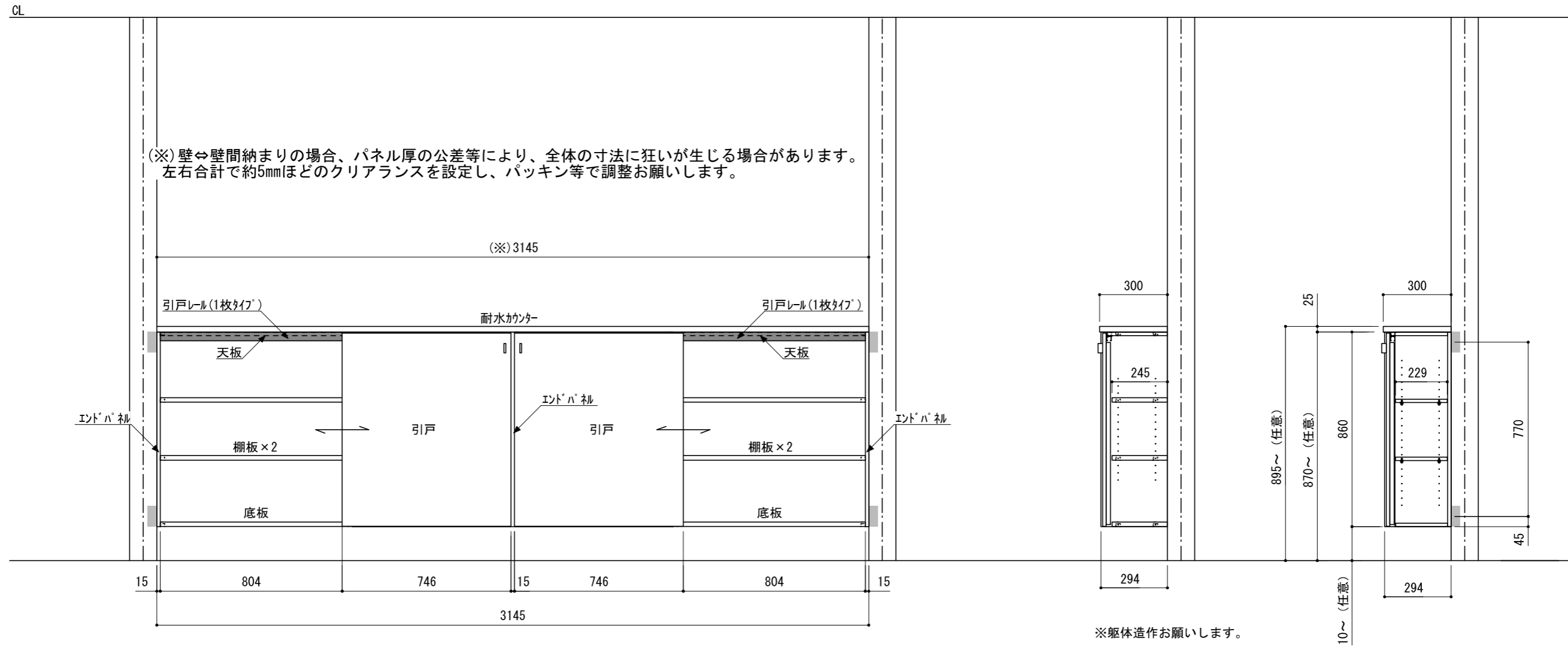
A-A' 断面
