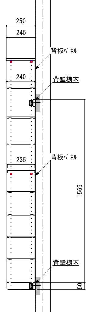
A-A' 断面
