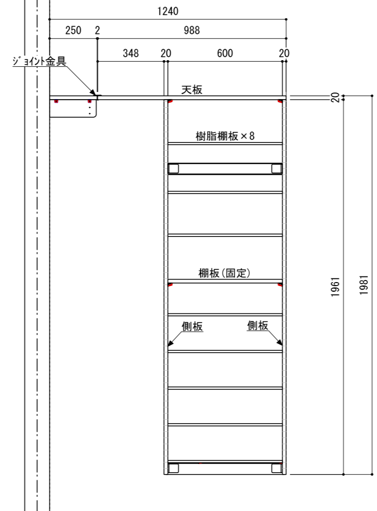
B-B' 断面
