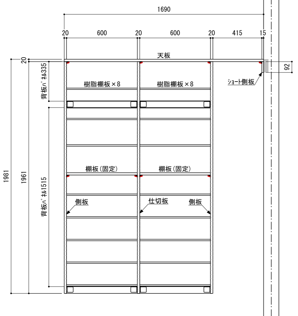
A 立面
