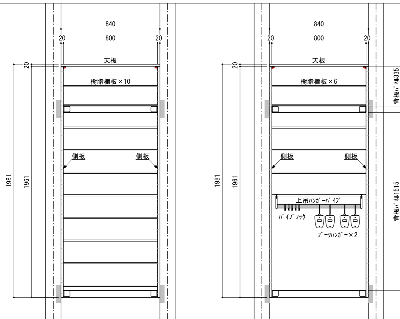
A 立面
