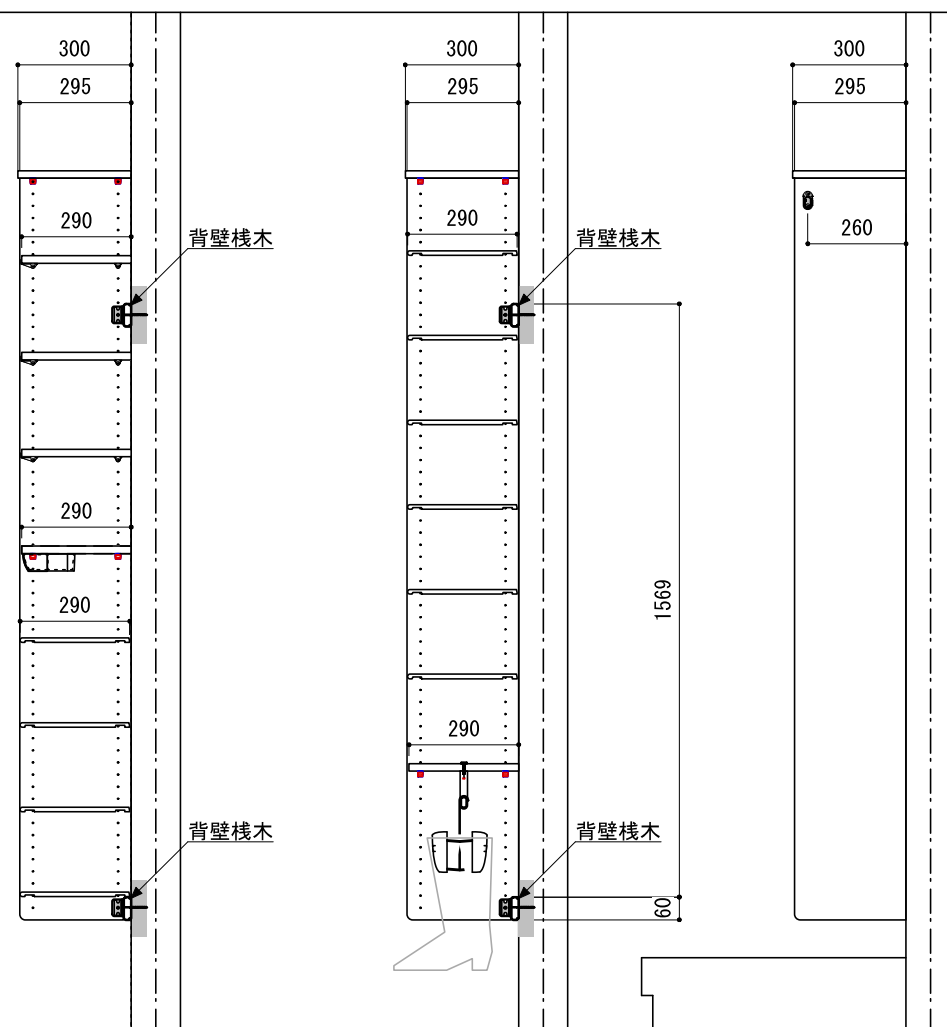
A-A' 断面
