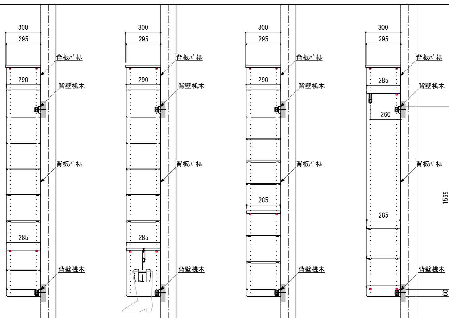
A-A' 断面
