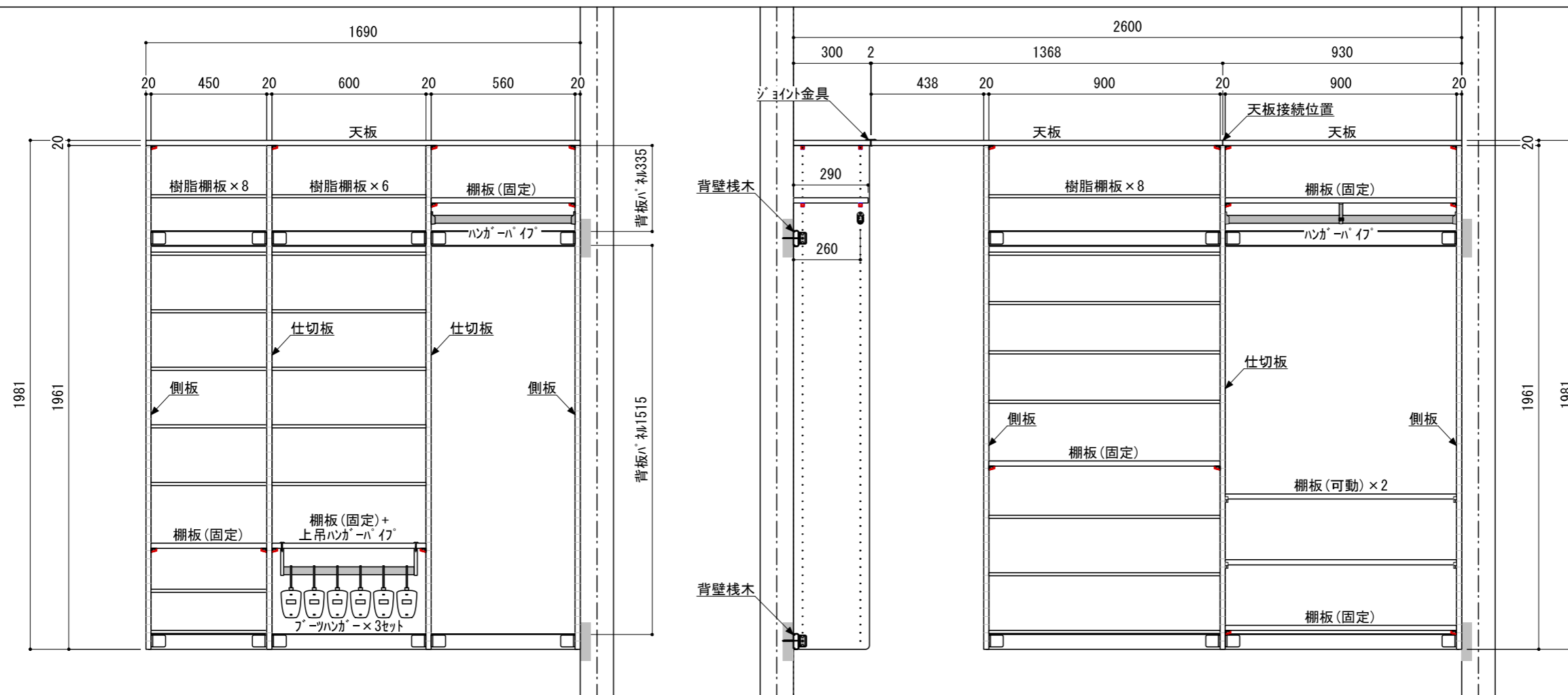
C-C' 断面
