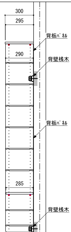
B-B' 断面
