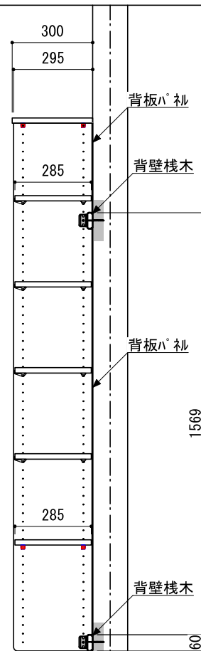
D-D' 断面
