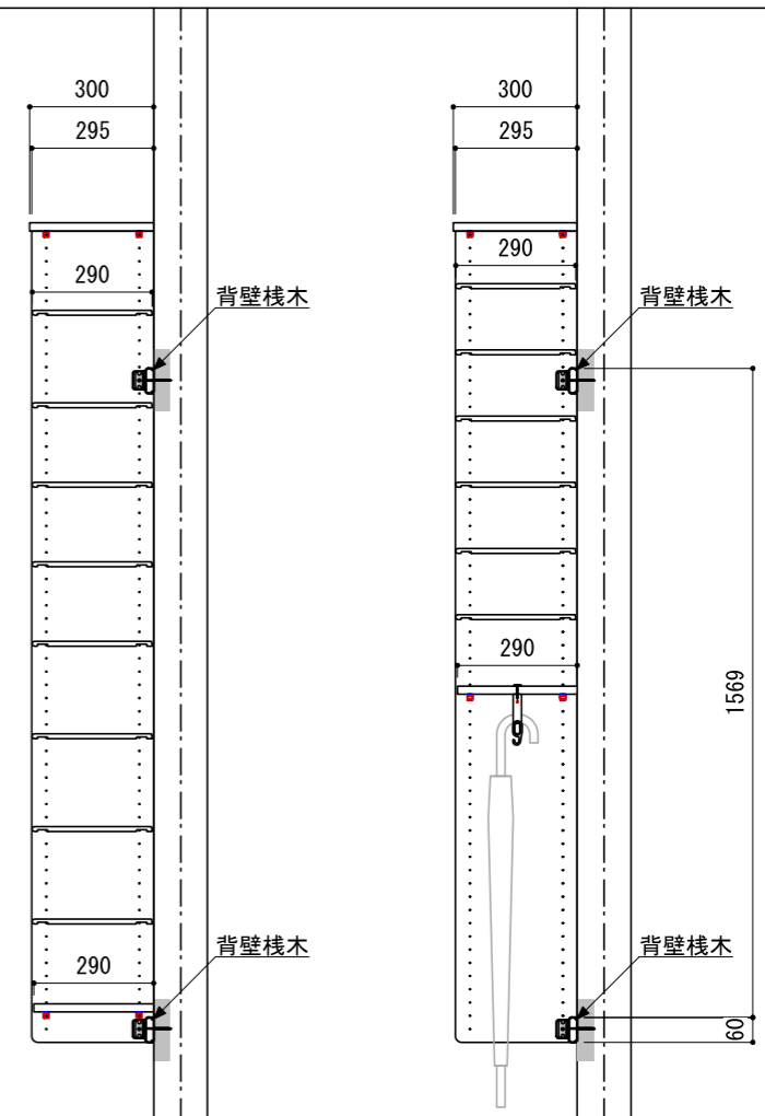
A-A' 断面
