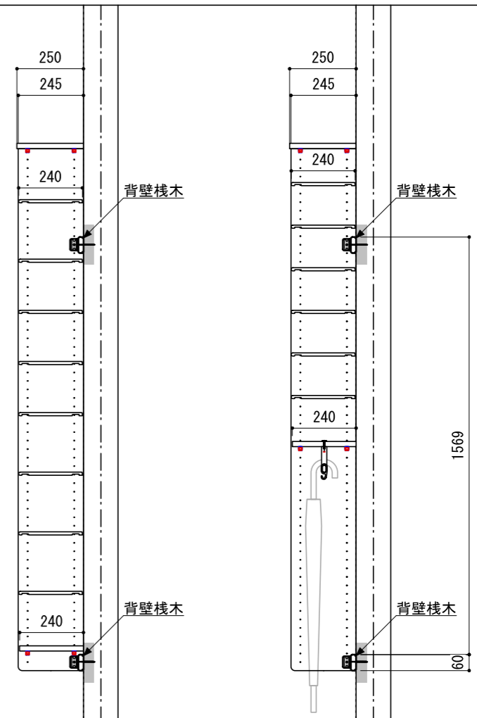
A-A' 断面
