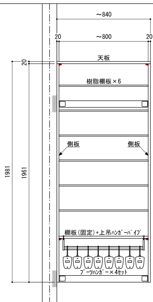
C立面
