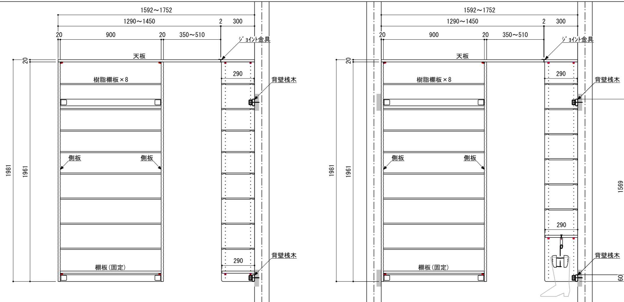
A-A' 断面
