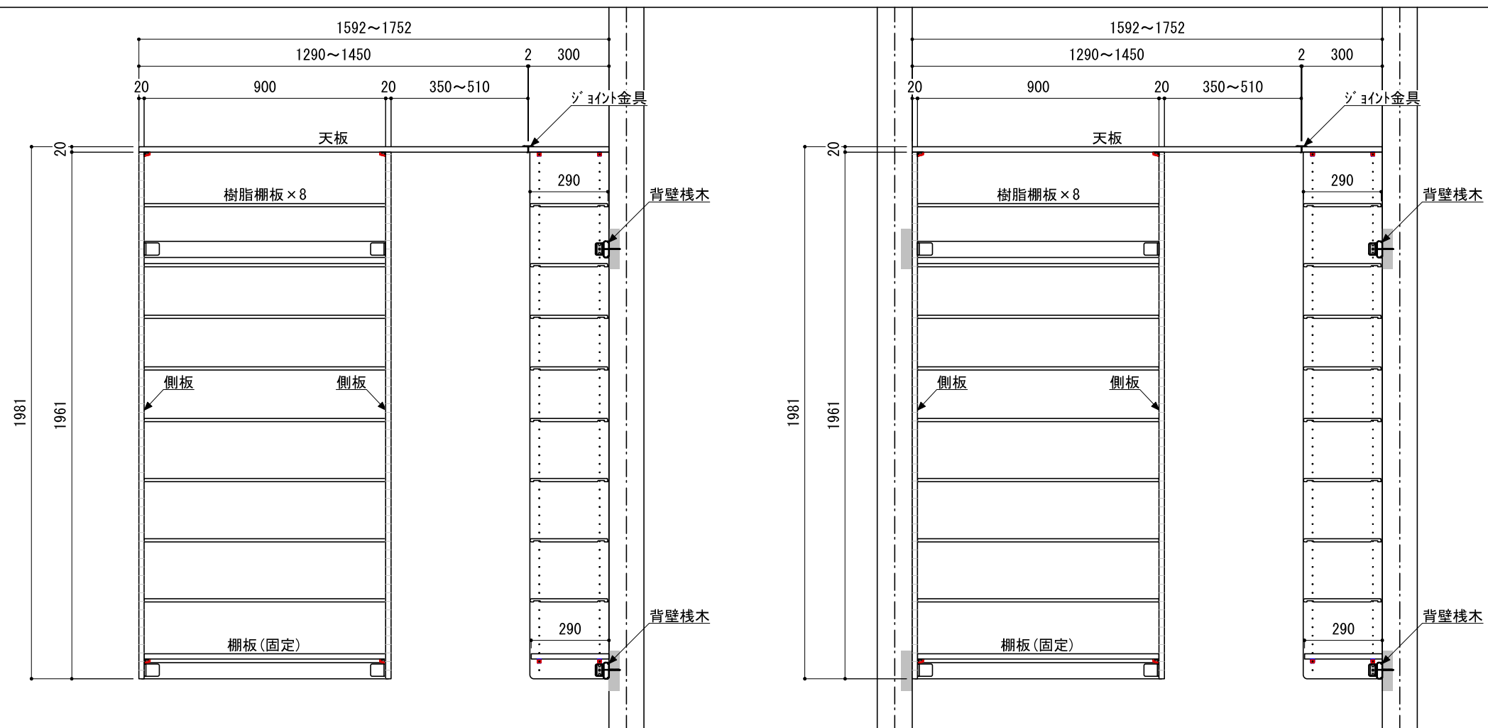
A 立面
