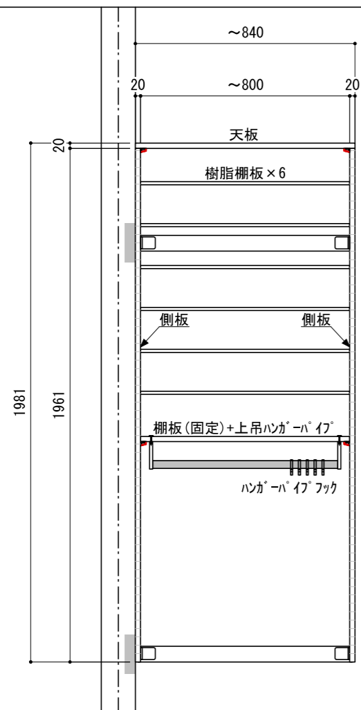
○ 立面
