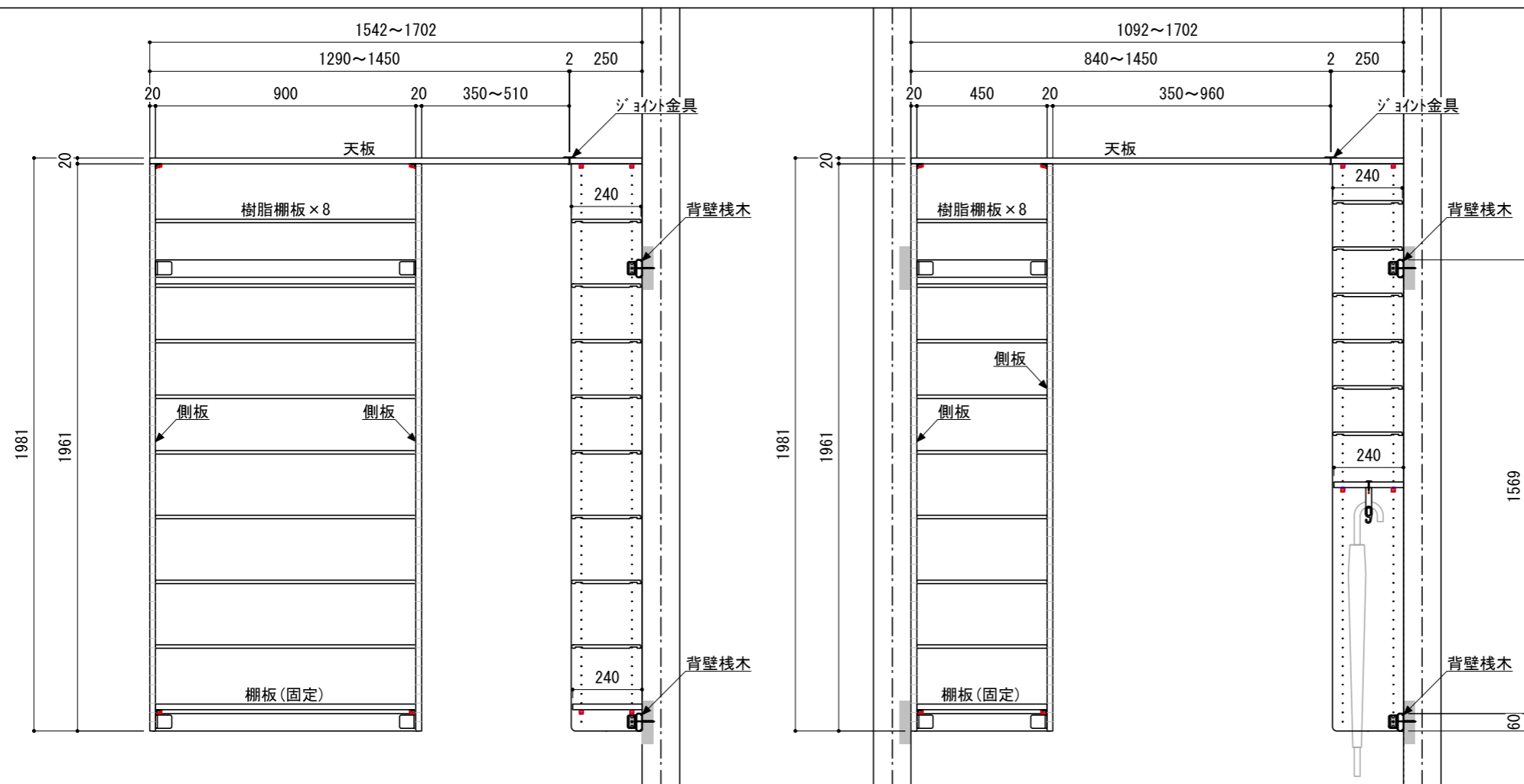
A 立面
