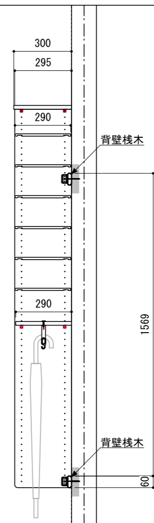
C-C'断面
