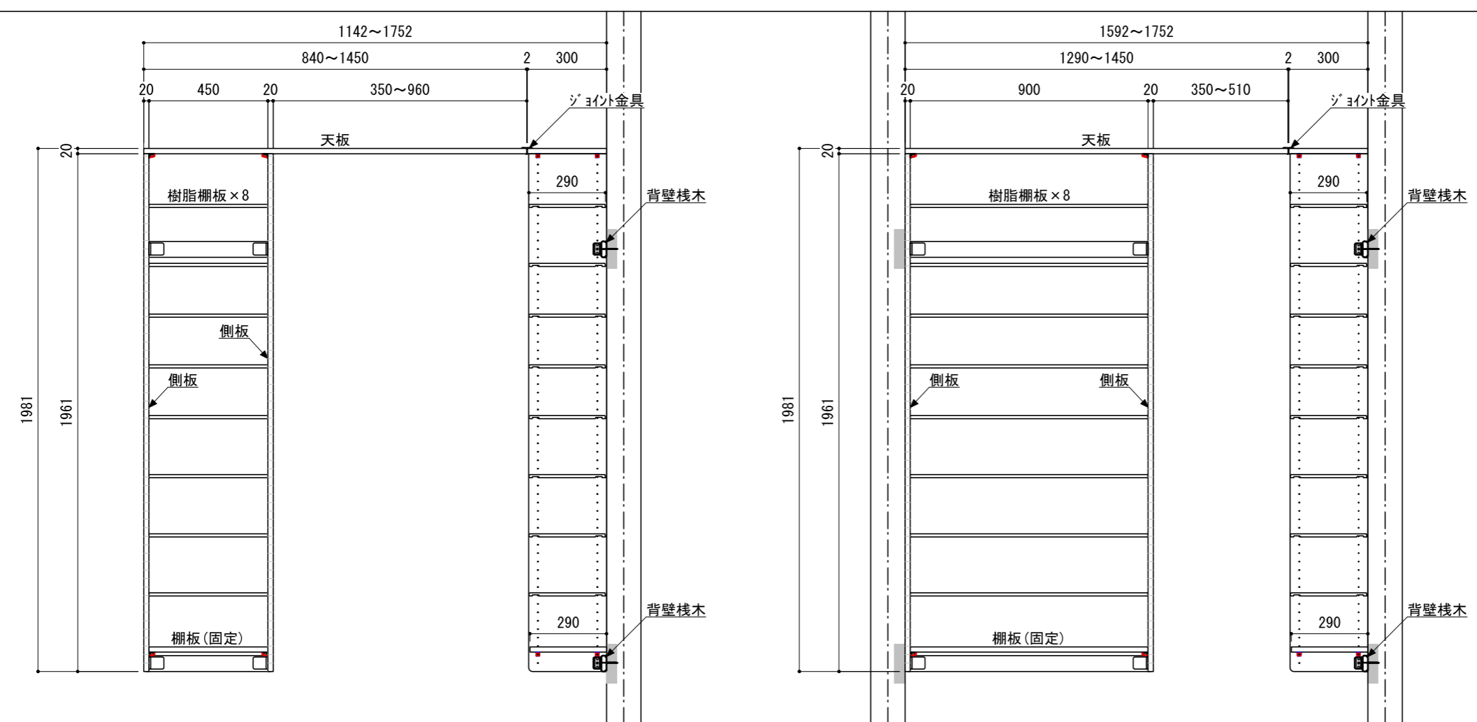
A立面
