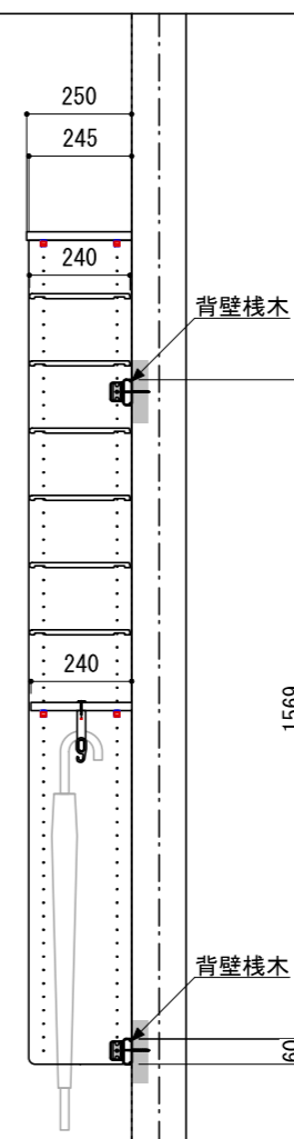
C-C'断面
