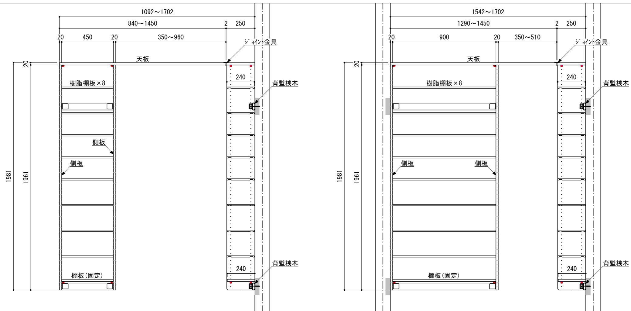
A 立面
