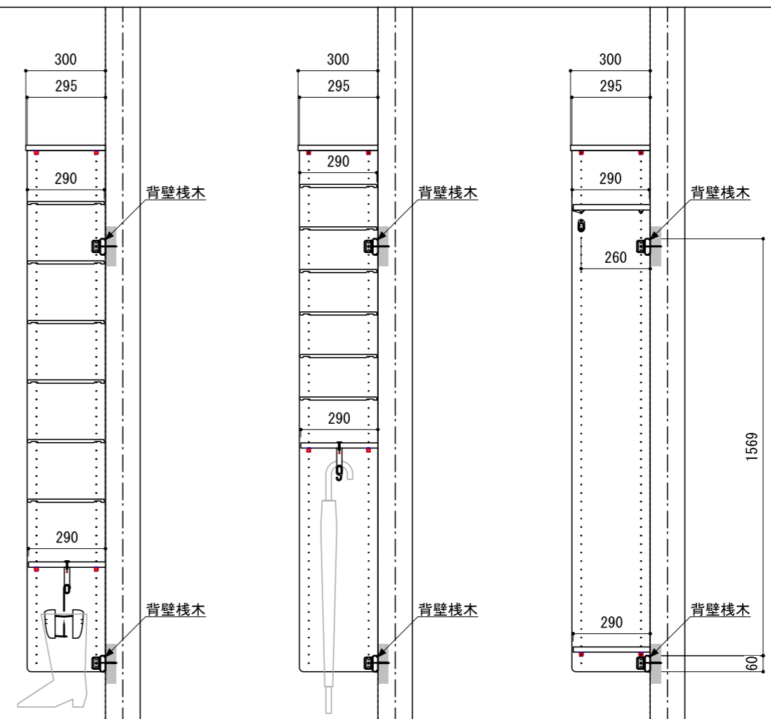
A-A' 断面
