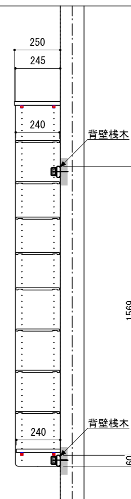
A-A' 断面
