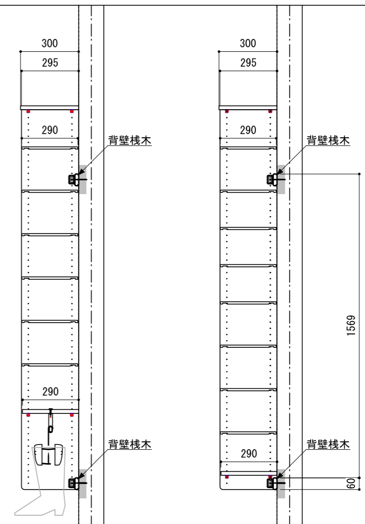
A-A' 断面
