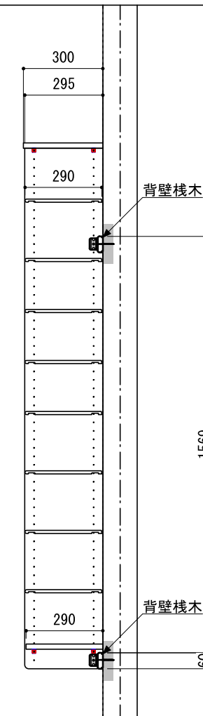
A-A' 断面
