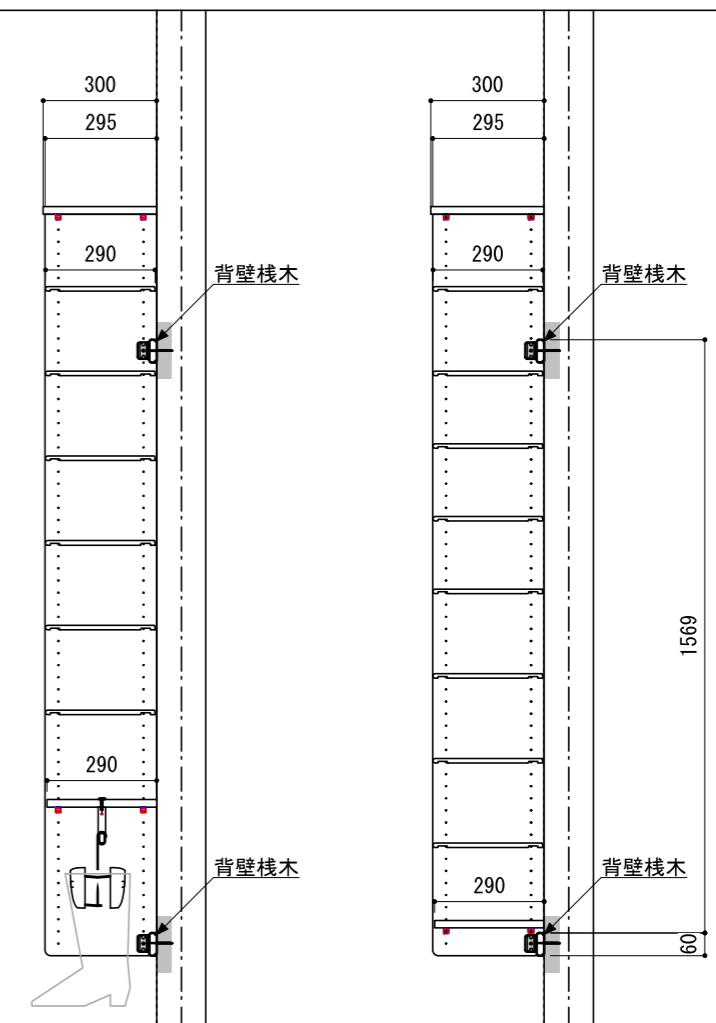
A-A' 断面
