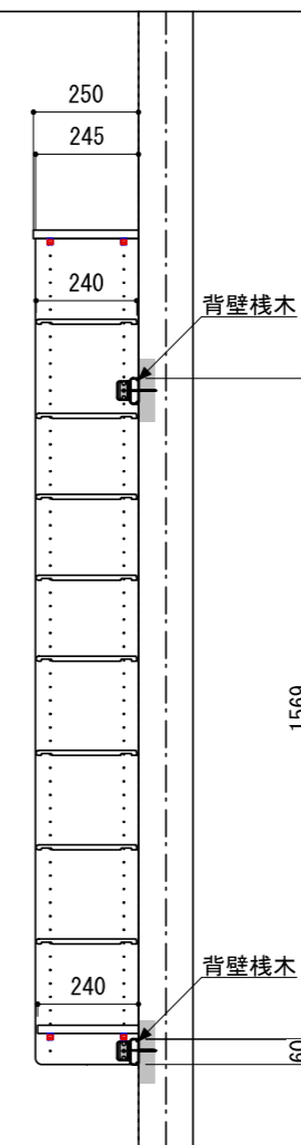
A-A' 断面
