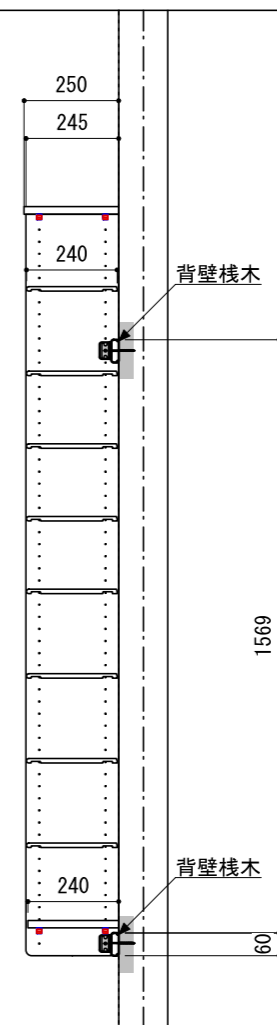
A-A' 断面
